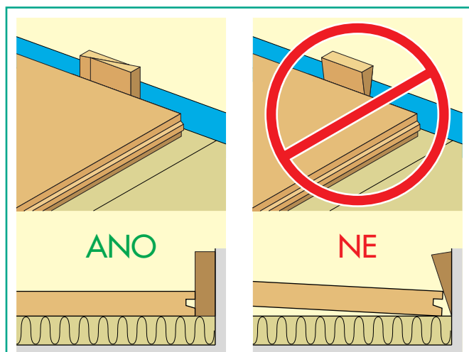
Způsob klínování obvodových dilatačních spár
