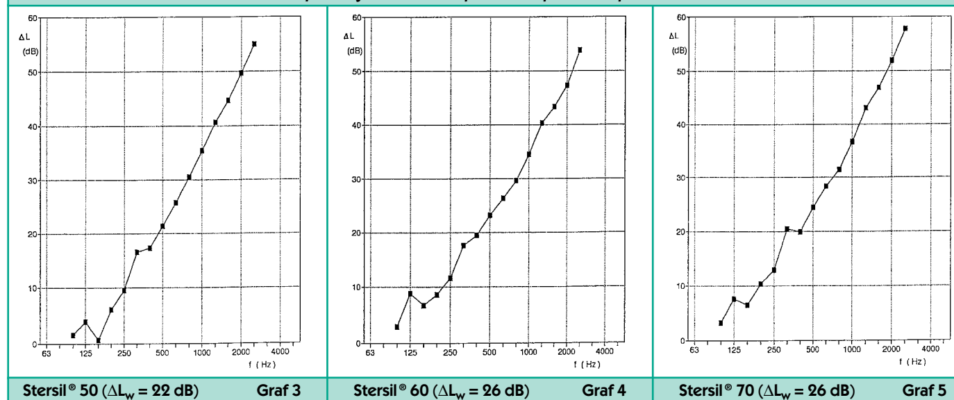
Průběh změny kročejového zvuku způsobené podlahou podle ČSN 73 05 18
